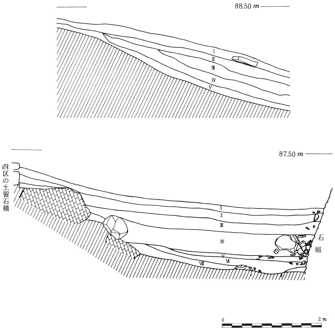
第55図 第5区北壁断面図（上は第4区の北側、下は第4区から第5区。場所は若干ちがうが、上図から下図へほぼ繋がる）
