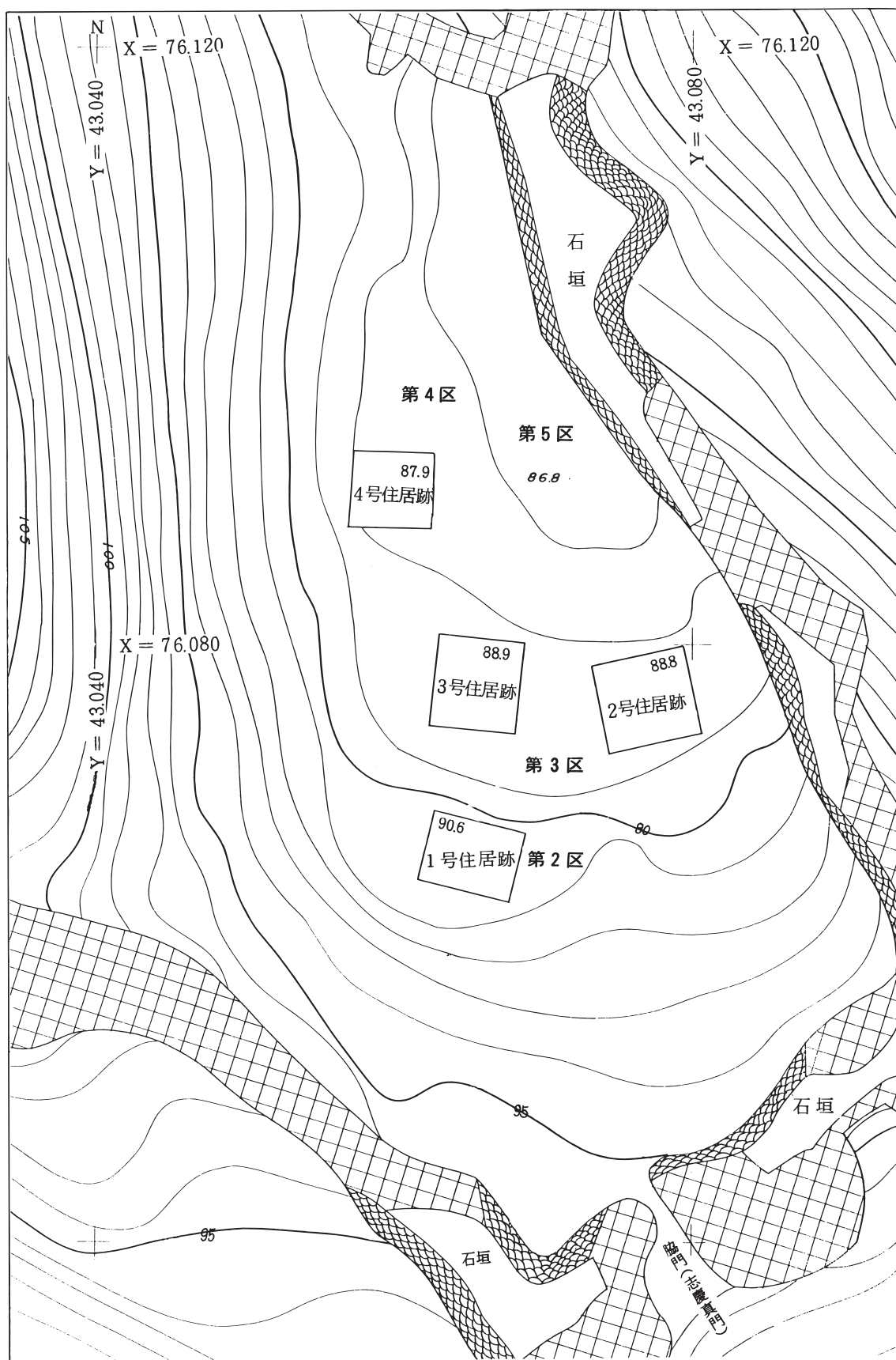
第54図 志慶真門郭の地形図 (1 : 400)
