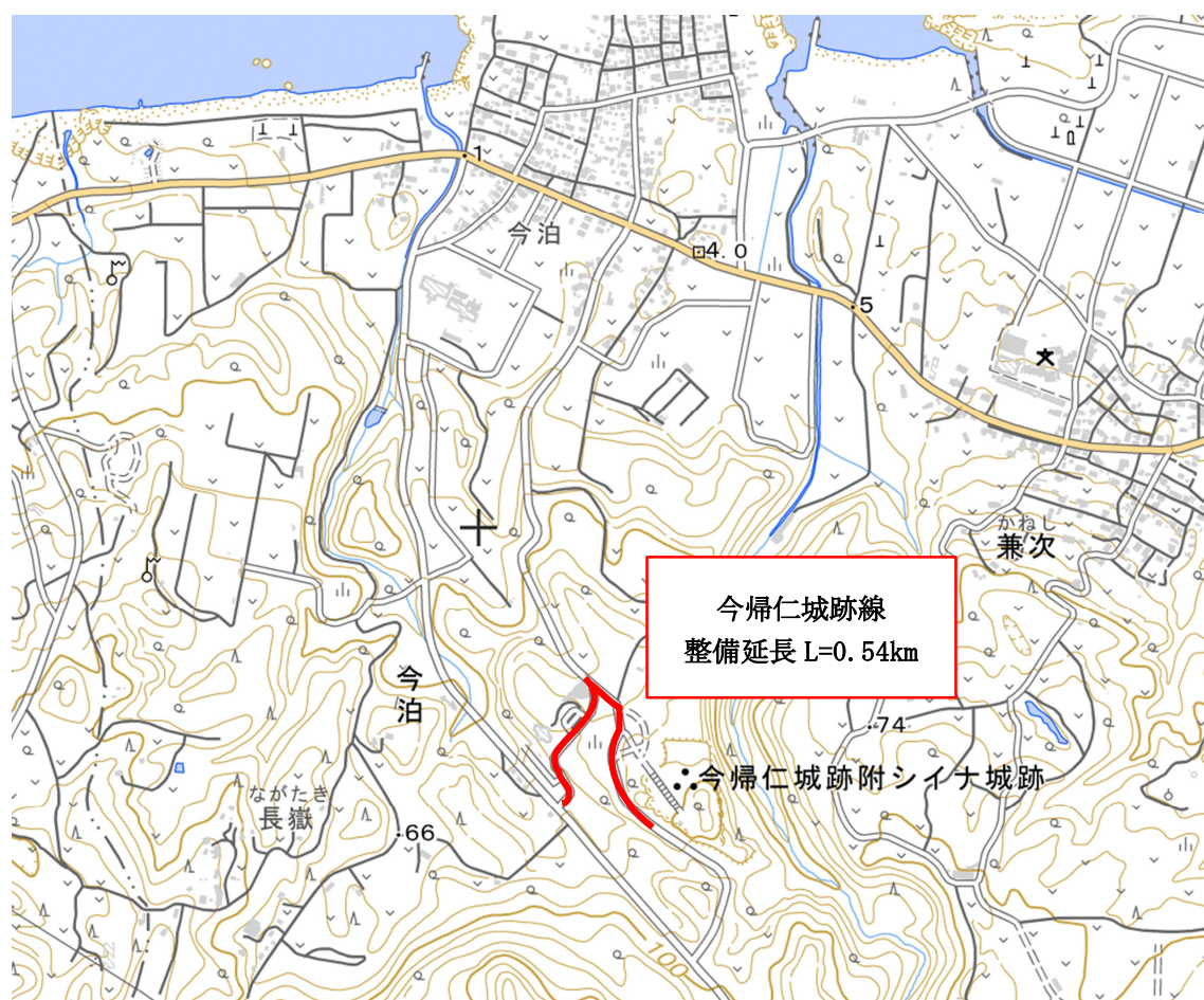
図-2 無電柱化計画路線位置図
