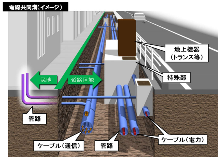
図ー4 電線共同溝イメージ図(出典:国土交通省HP)
