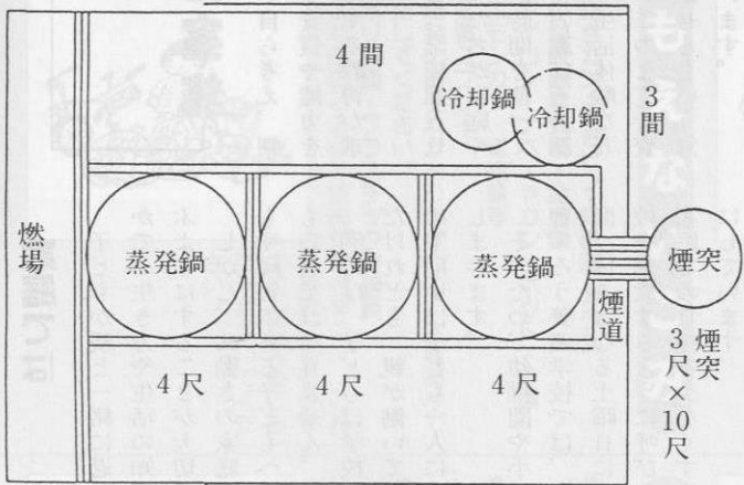
▲砂糖屋の平面図(『諸志共同組合のあゆみ』より)
