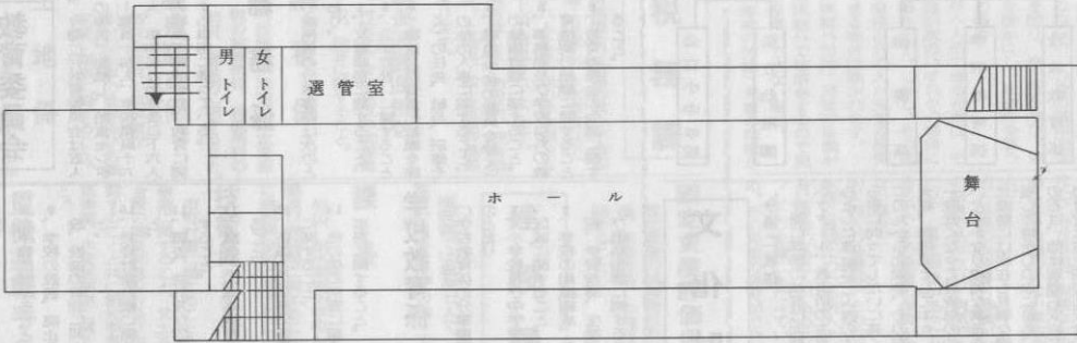
2 階 平 面 図
